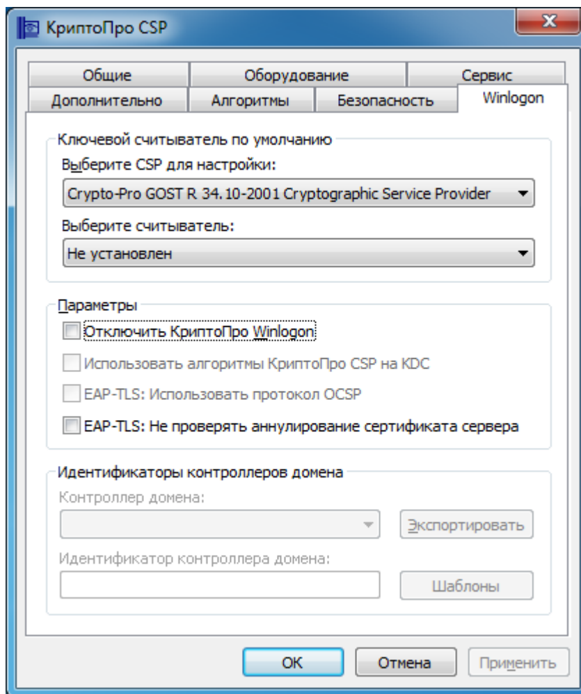
Рис. 65. Контрольная панель, вкладка Winlogon.
