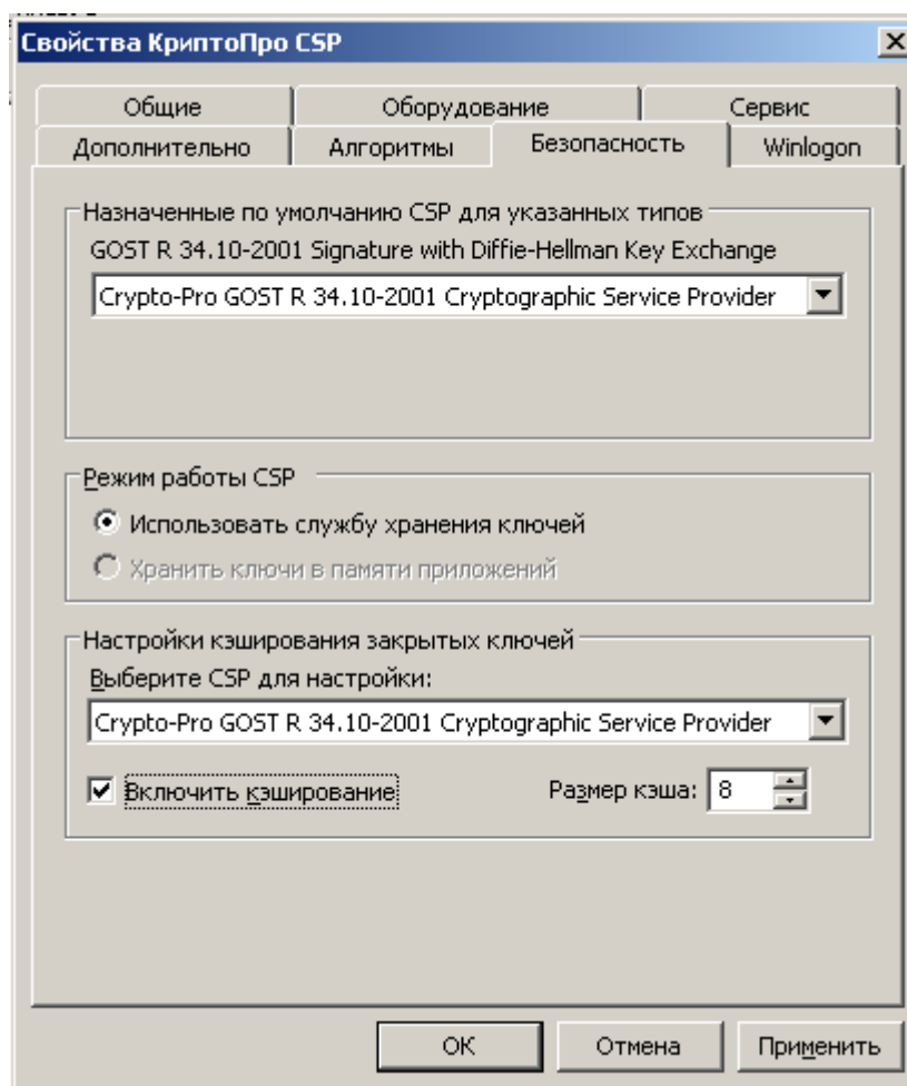
Рис. 60. Вкладка Безопасность, уровень защиты КС2.
